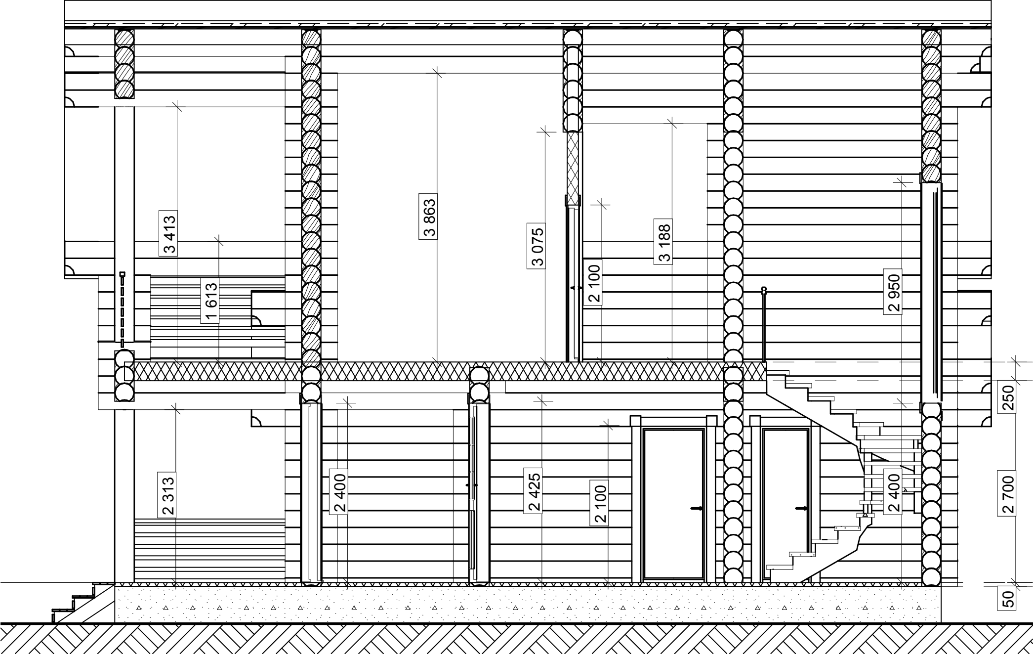
Разрез 1-1
