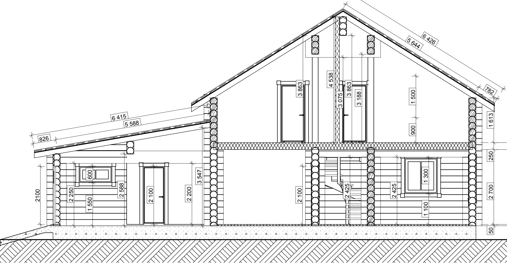
Разрез 2-2
