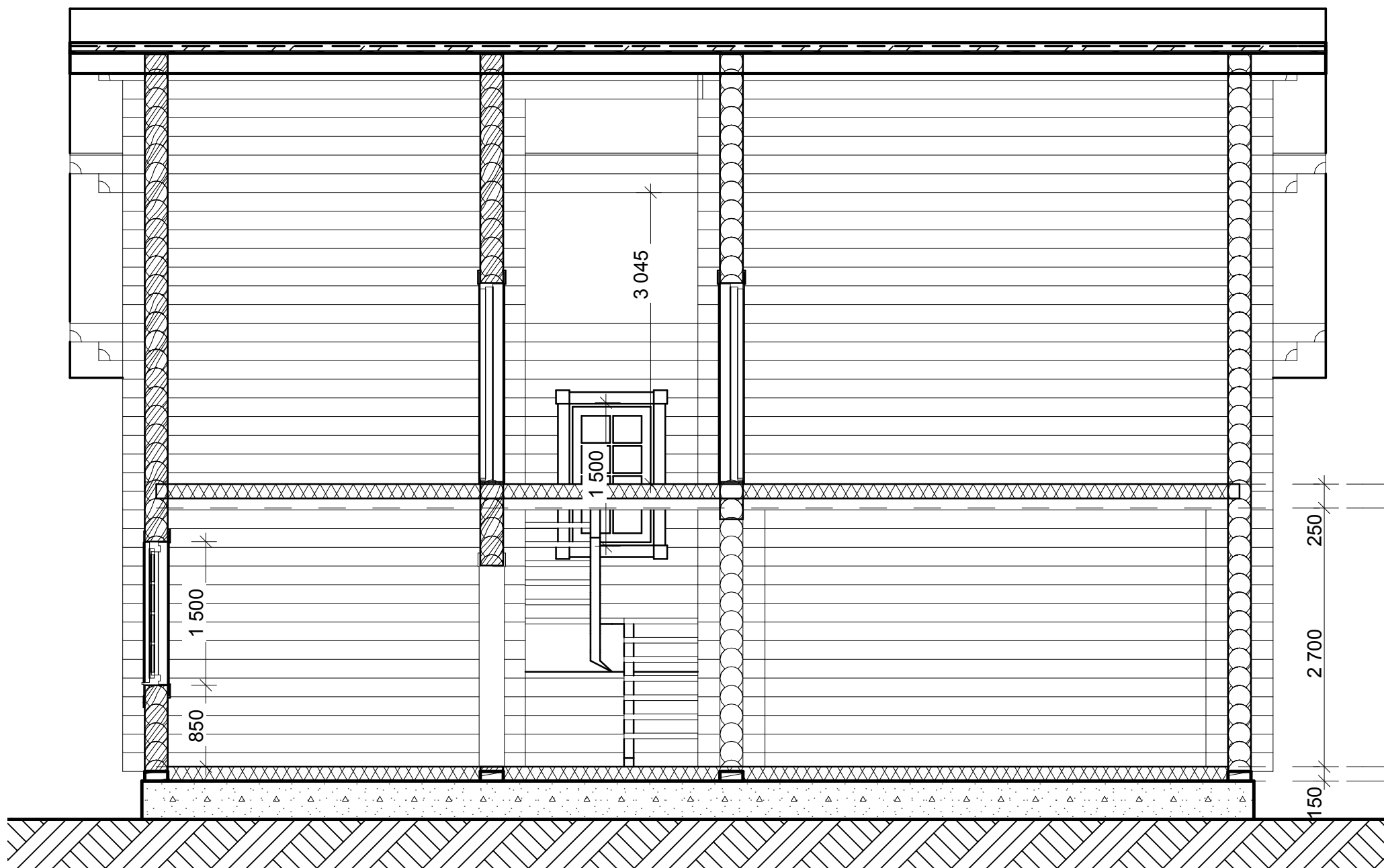
Разрез 2-2
